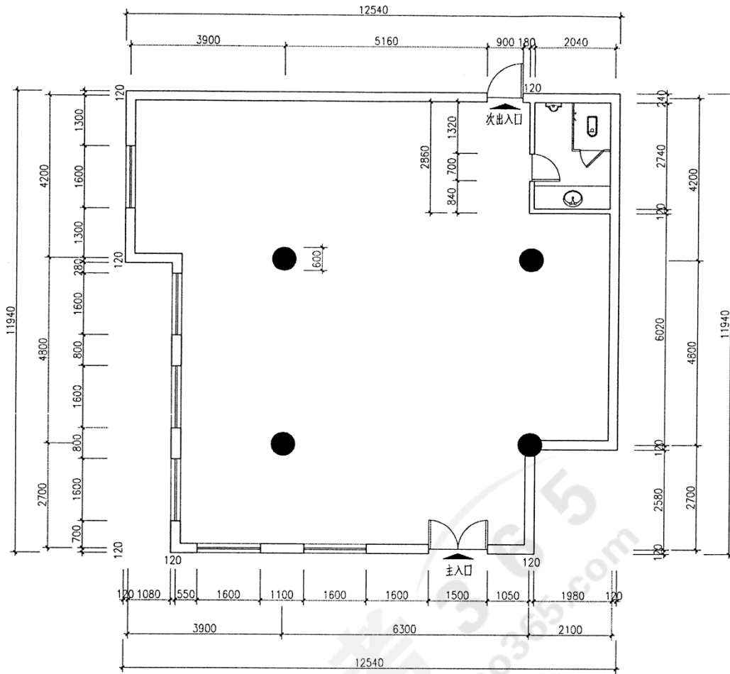
(尺寸参考图)
