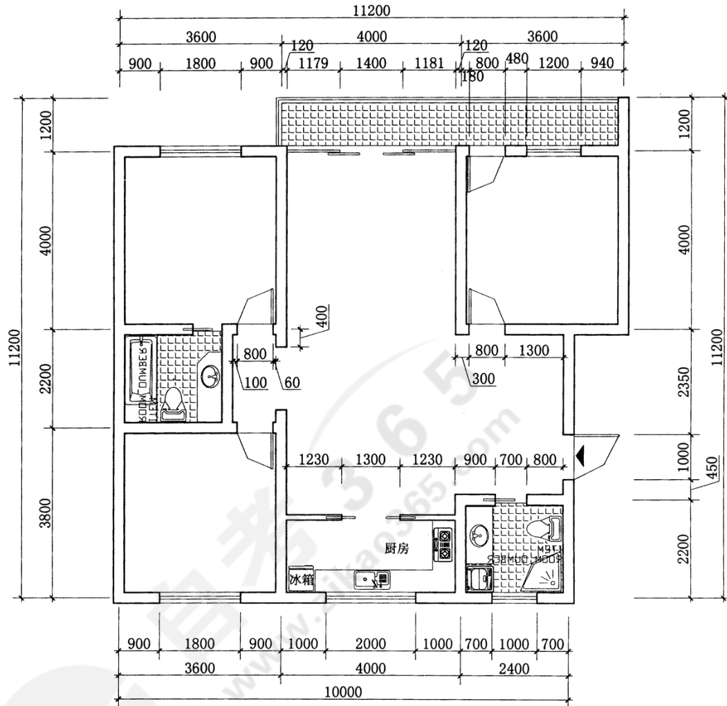
尺寸参考图
