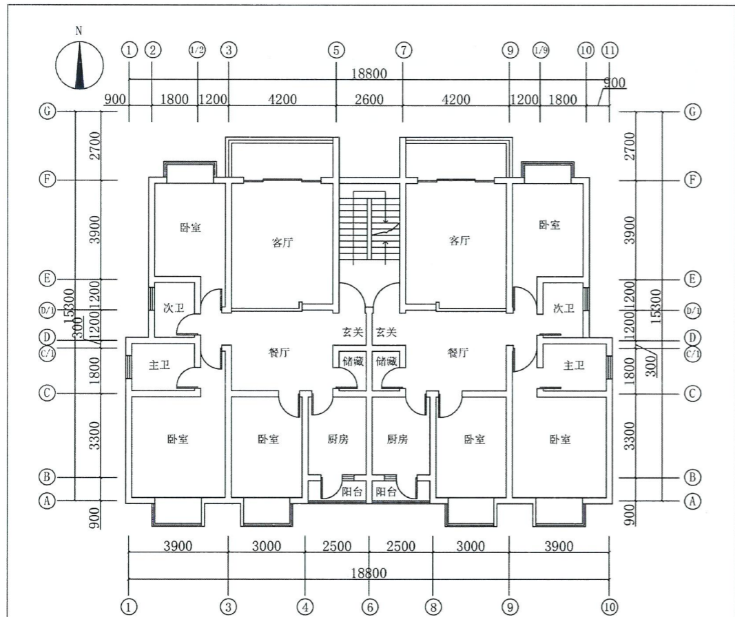
某建筑标准层平面图 1:200
