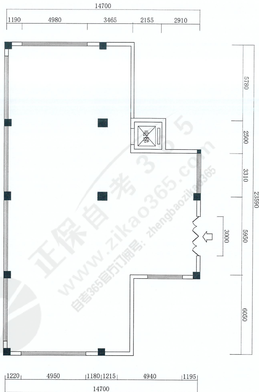
某冷饮吧室内平面图
