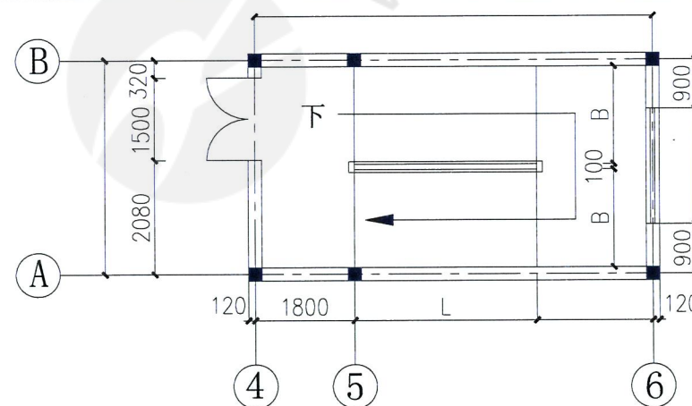
图 1 楼梯顶层平面图
