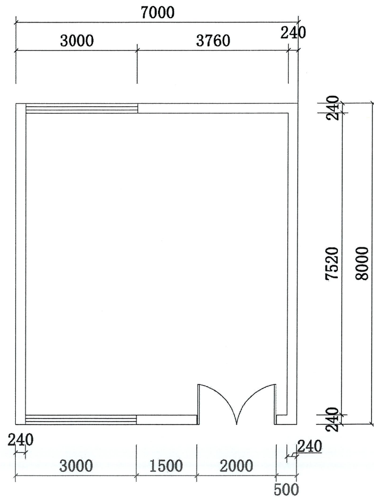
原始平面图 单位：mm
