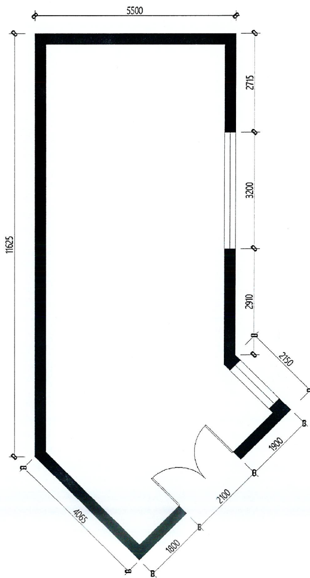
原始平面图 (单位: mm)
