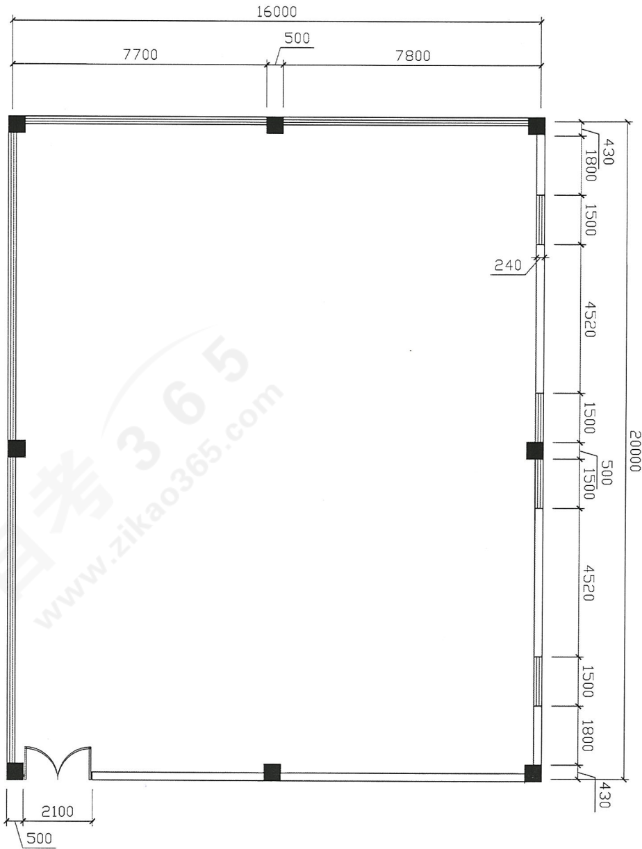
某火锅店室内平面图（单位：mm）
