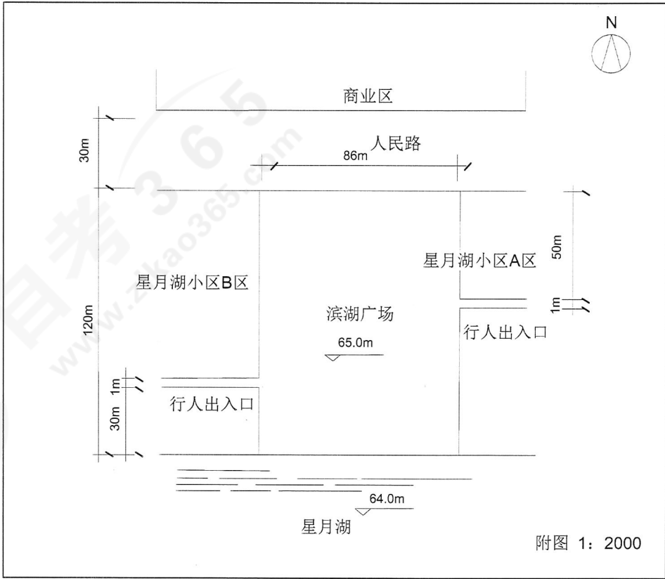
滨湖广场基址平面图
