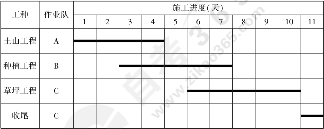
图 1 某园林工程施工进度计划横道图
