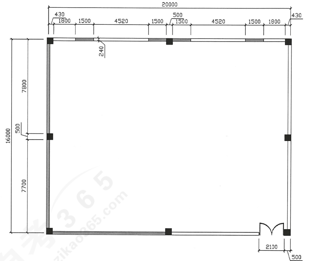
某网红奶茶店室内设计（单位：mm）
