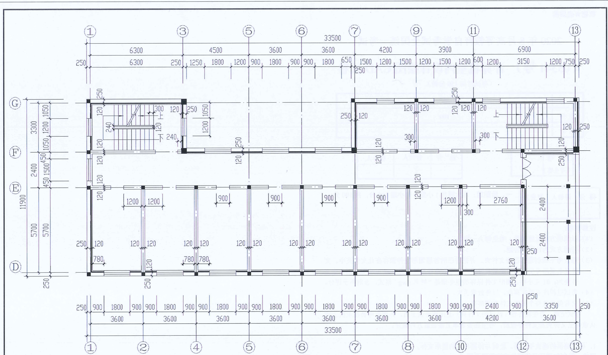
某住宅建筑平面图 1:100
