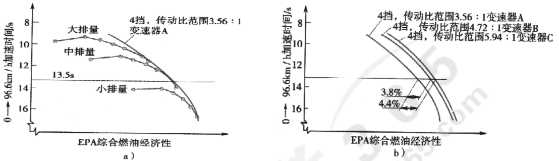
(题 41 图)不同排量发动机与不同变速器的最佳燃油经济性和动力性曲线
